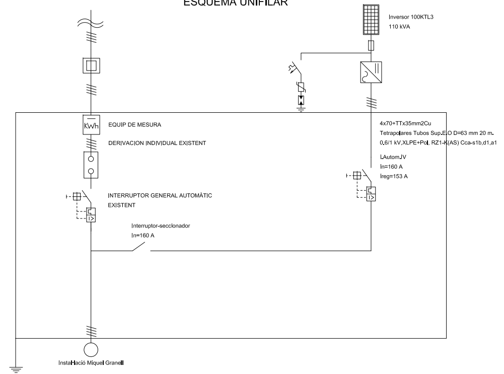
ESQUEMA UNIFILAR
