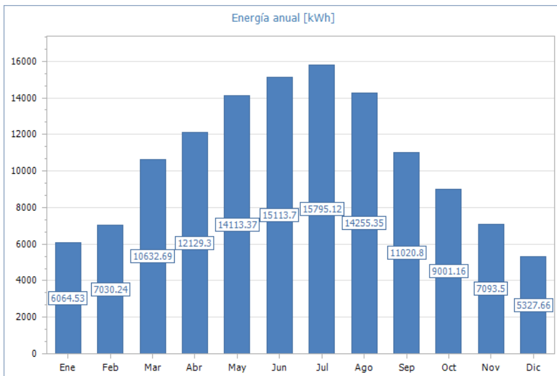
Fig. 3: Energia mensual produïda per la instal·lació
