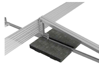
Ejemplo de instalación de 2 contrapesos de 1de hasta 200 mm de ancho repartidos sobre portalastre.
