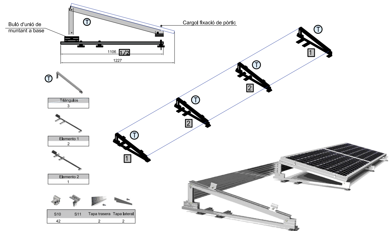
ESTRUCTURA DE SUPORT INCLINADA LASTRADA PER A COBERTA PLANA 29H - Col·locació horitzontal - 1 fila 3 mòduls
