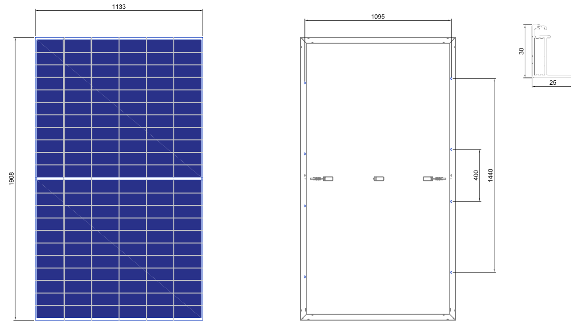
MÒDUL SOLAR SUNRISE SR-60M450HLPRO o similar
