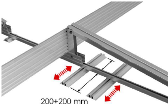
Regulación del portalastre (Ejemplo colocación de portalastre centrado).
