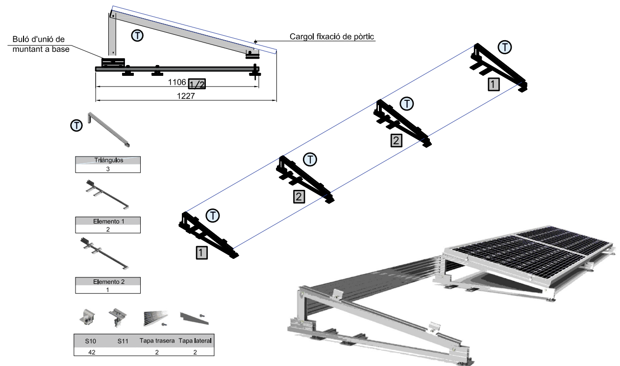
ESTRUCTURA DE SUPORT INCLINADA LASTRADA PER A COBERTA PLANA 29H - Col·locació horitzontal - 1 fila 3 mòduls
