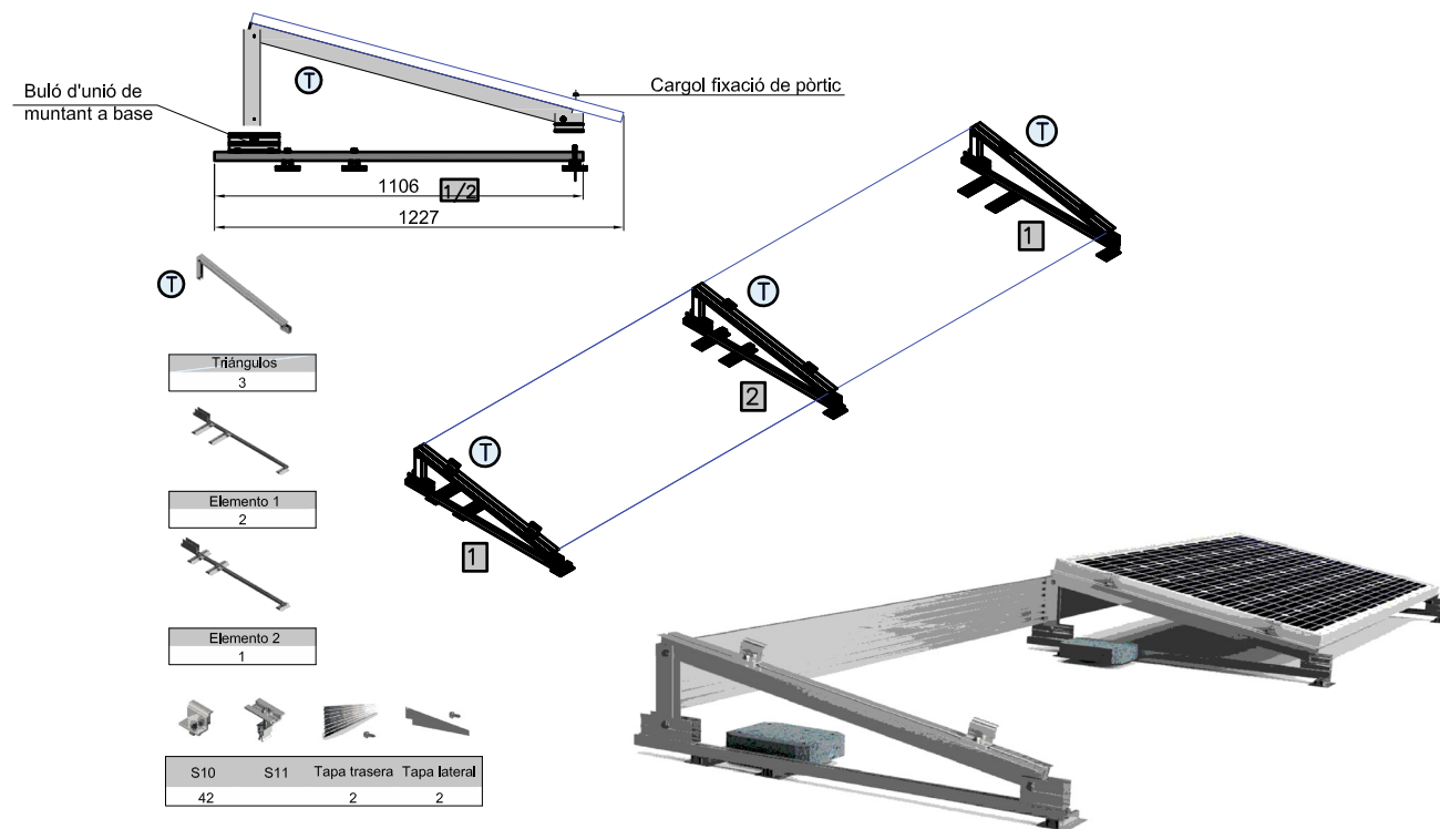
ESTRUCTURA DE SUPORT INCLINADA LASTRADA PER A COBERTA PLANA 29H - Col·locació horitzontal - 1 fila 2 mòduls
