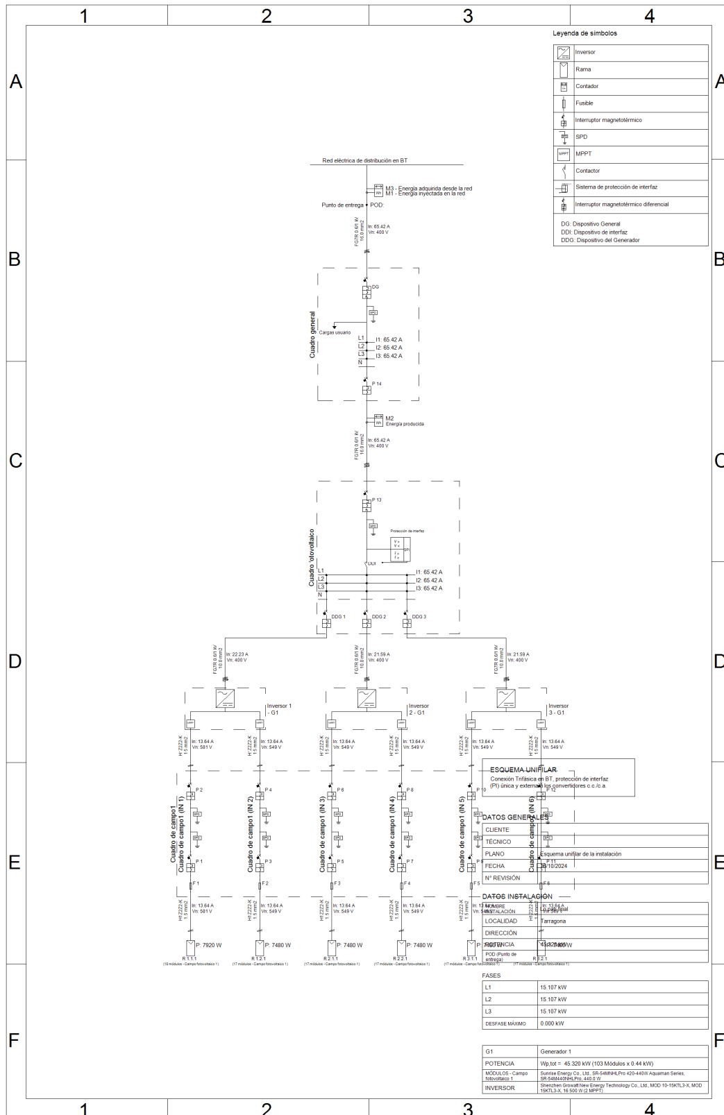
Fig. 8: Esquema elèctric unifilar de la instal·lació
